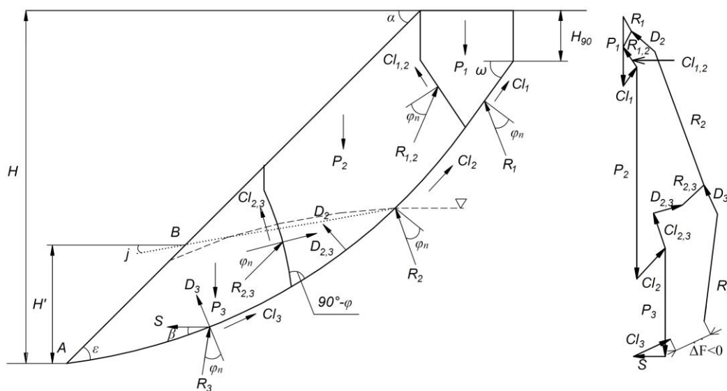
Рисунок 3 – Схема расчёта устойчивости обводнённого изотропного откоса с учётом воздействия сейсмических сил методом векторного сложения сил: P_i – вес рассматриваемого блока, мН; Cl_{i,i+1} , Cl_{i,i-1} , Cl_i – силы сцепления, направленные параллельно соответствующим границам блоков, мН; D_{i,i+1} , D_{i,i-1} , D_i – силы гидростатического давления по границам блоков, мН; R_{i,i+1} , R_{i,i-1} , R_i – реакции по границам блоков, мН; S – сейсмическая сила, мН; \beta – угол наклона сейсмической силы, град.
