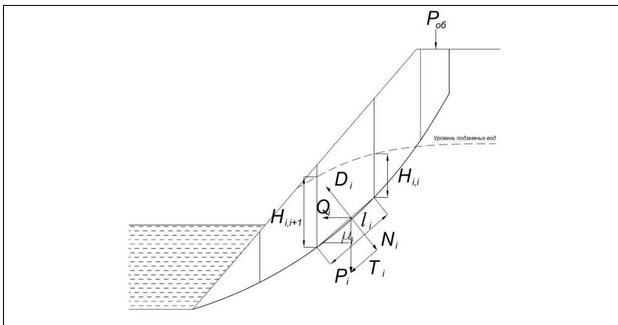
Рисунок 2 – Расчет устойчивости обводненного изотропного откоса с учетом воздействия сейсмических сил методом алгебраического сложения сил
