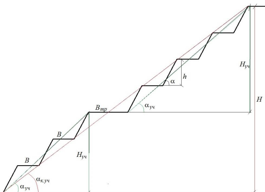
Рисунок 1. Схема конструкции бортов и уступов: h , H_{уч} , H – соответственно высота уступа, групп уступов, борта; \alpha_{уч} , \alpha_{к.уч} , \alpha – соответственно, угол откоса уступа, конструктивной группы уступов и борта карьера, разреза; B , B_{mp} – соответственно, ширина предохранительной и транспортной бермы
